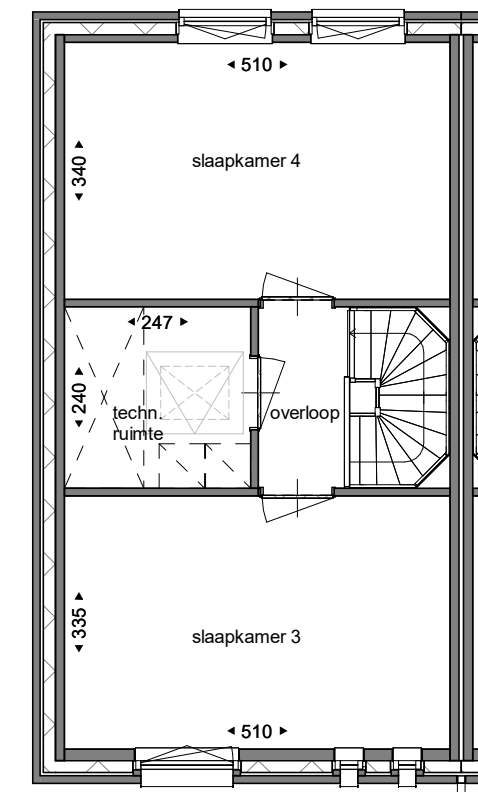
tweede verdieping
