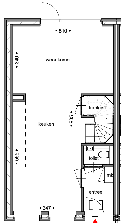
begane grond
