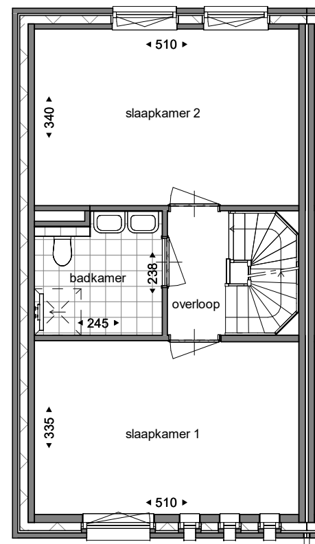
eerste verdieping
